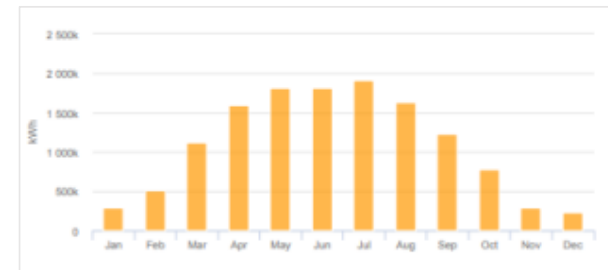
Prognostizierte Erträge in kWh nach Monaten. Es werden über 3.000 Haushalte mit Strom versorgt werden können.
